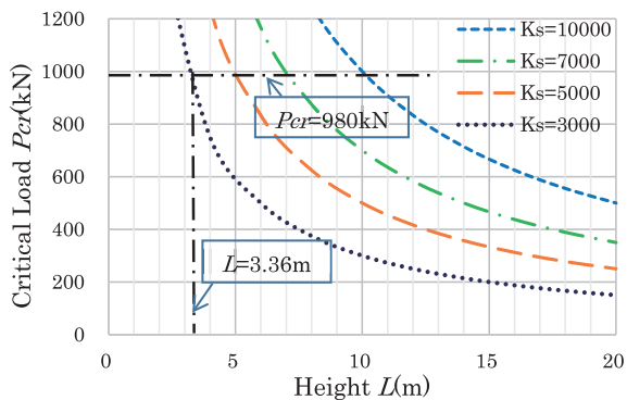
図4 転倒荷重-限界高さ関係
