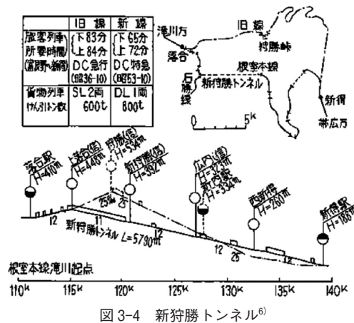
図 3-4 新狩勝トンネル 6)
