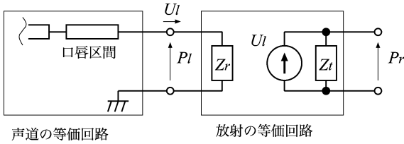
図1 放射過程の等価回路
