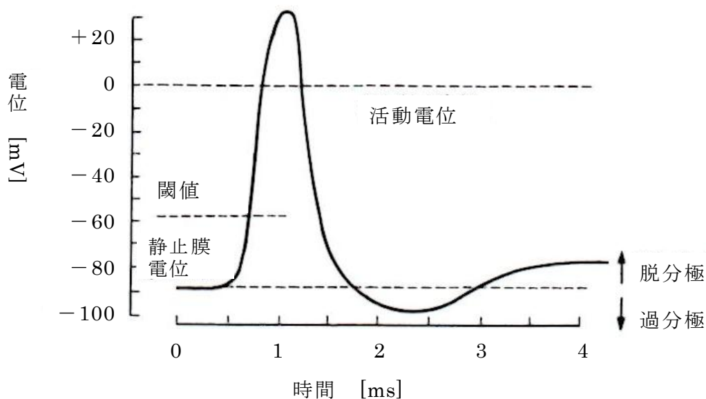
図 2.14 活動電位 [9]
