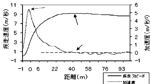
図 1 100 m 走における疾走速度曲線および、加速度の変化
