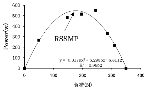
図14 負荷とパワーの関係
